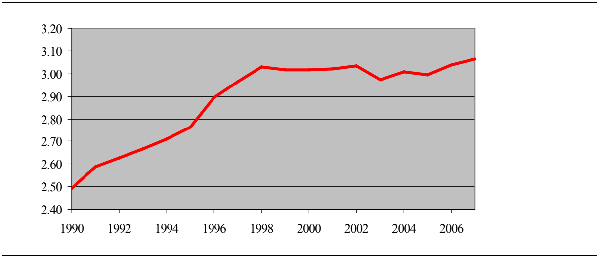
Abb. 3-25: Entwicklung der JAZ für Luft-Wasser-Wärmepumpen anhand der für die FAWA ausgewählten Wärmepumpen (96 Anlagen)
