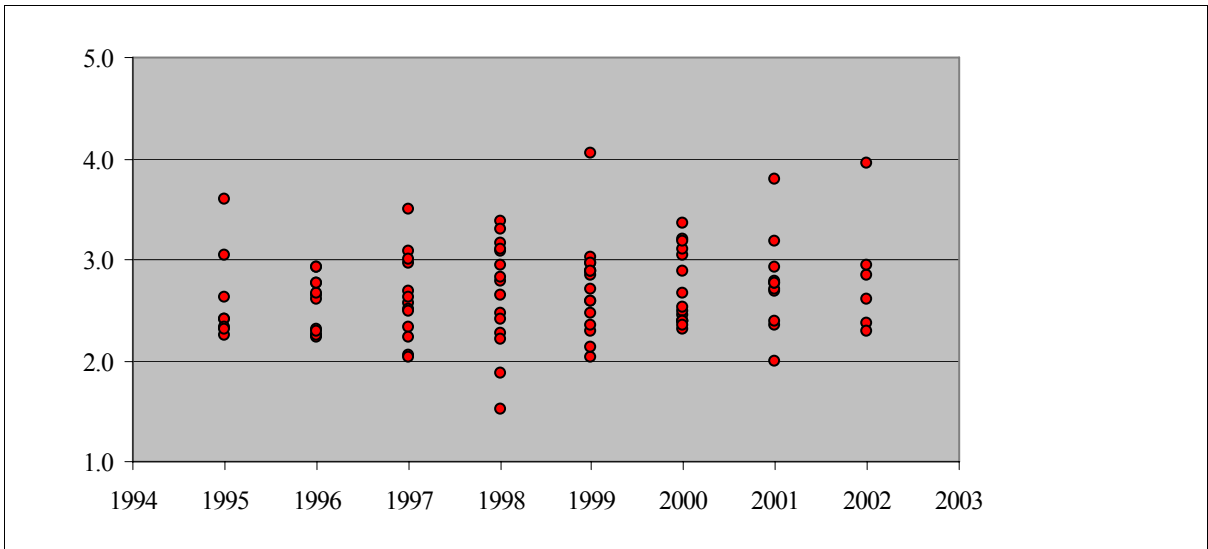
Abb. 3-25: Entwicklung der JAZ für Luft-Wasser-Wärmepumpen anhand der für die FAWA ausgewählten Wärmepumpen (96 Anlagen)
