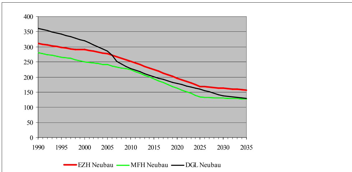
Abb. 3-20 Spezifischer Heizenergieverbrauch für Neubauten (MJ pro m 2 , Quellen: Prognos, CEPE)
