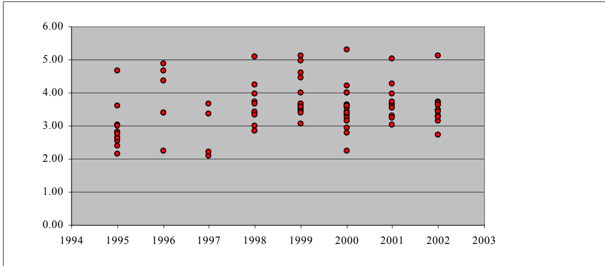
Abb. 3-26: Entwicklung der JAZ für Sole-Wasser-Wärmepumpen anhand der für die FAWA ausgewählten Wärmepumpen (86 Anlagen)
