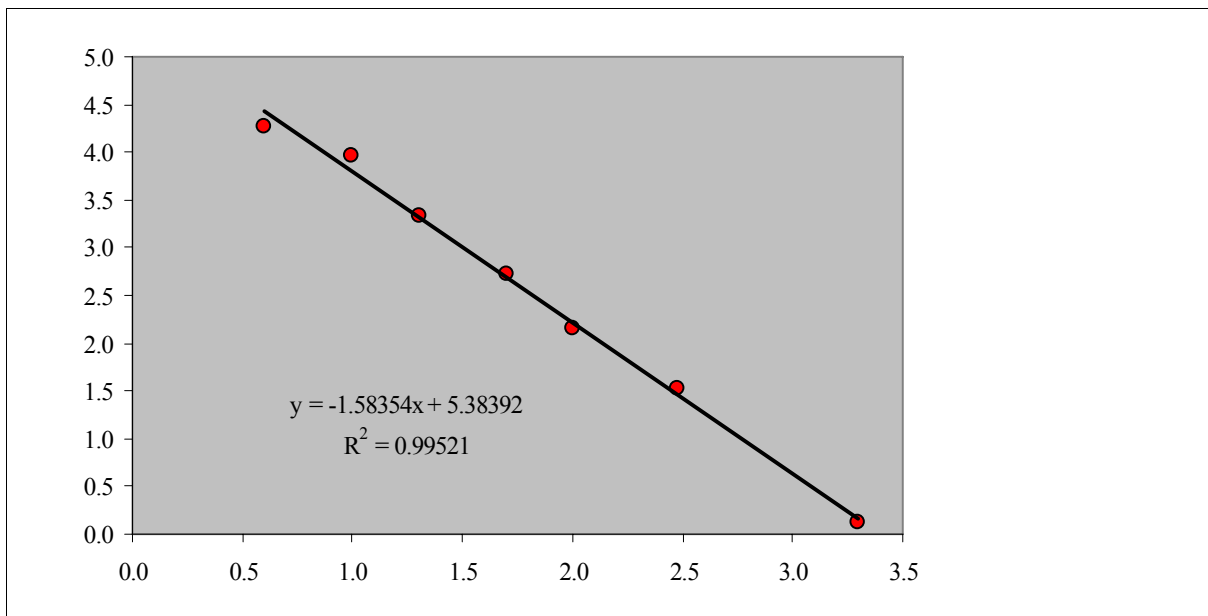
Abb. 3-23: Verteilung der Leistungen für Sole/Wasser-Wärmepumpen (eingetragen sind nicht die x- und y-Werte selbst, sondern deren Zehnerlogarithmen)
