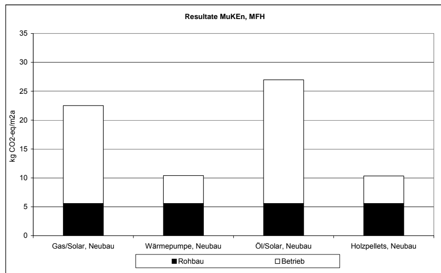
Abbildung 28: Treibhauspotential (in kg CO 2 -eq/m 2 a) für Bau, Betrieb und Rückbau von Mehrfamilienhäusern nach MuKE Modul 2 für Neubauten. Der Anteil Rohbau (ohne Wärmedämmung) ist separat ausgewiesen.
