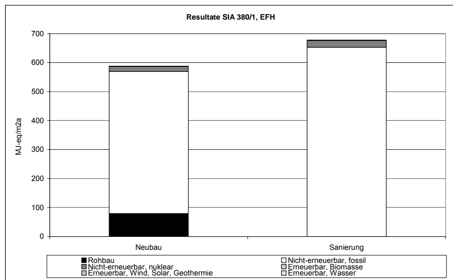
Abbildung 14: Kumulierter Energieaufwand (in MJ-eq/m 2 a) für Bau, Betrieb und Rückbau von Einfamilienhäusern nach SIA 380/1 Grenzwert für Neubau bzw. Sanierung. Der Anteil Rohbau (ohne Wärmedämmung) ist separat ausgewiesen.
