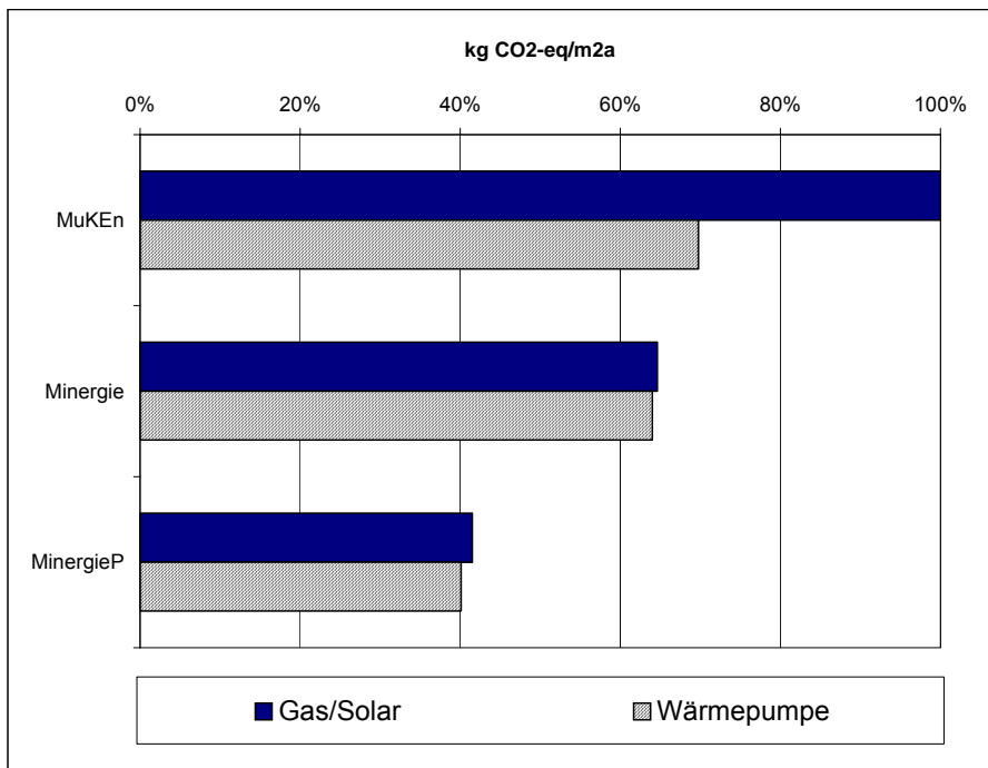
Abbildung 64: Vergleich des Treibhauspotentials 100a der Varianten Gas/Solar und Wärmepumpe (Einfamilienhaus, Neubau) beim Betrieb mit GuD-Strom. Die Variante MuKE n-M2, Gas/Solar wird zu 100% gesetzt und das Treibhauspotenzial der anderen Varianten und Standards dazu ins Verhältnis gesetzt.
