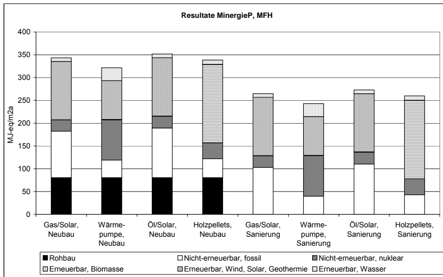
Abbildung 48: Kumulierter Energieaufwand, total (in MJ-eq/m 2 a) für Bau, Betrieb und Rückbau von Mehrfamilienhäusern nach Minergie-P für Neubauten und Sanierungen. Der Anteil Rohbau (ohne Wärmedämmung) ist separat ausgewiesen.
