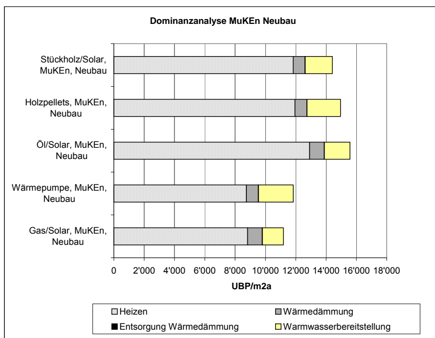
Abbildung 35: Bedeutung der verschiedenen Prozesse der Variante MuKEu-M2, Einfamilienhaus, Neubauten; bewertet mit der Methode der ökologischen Knappheit 2006 (provisorische Ökofaktoren).
