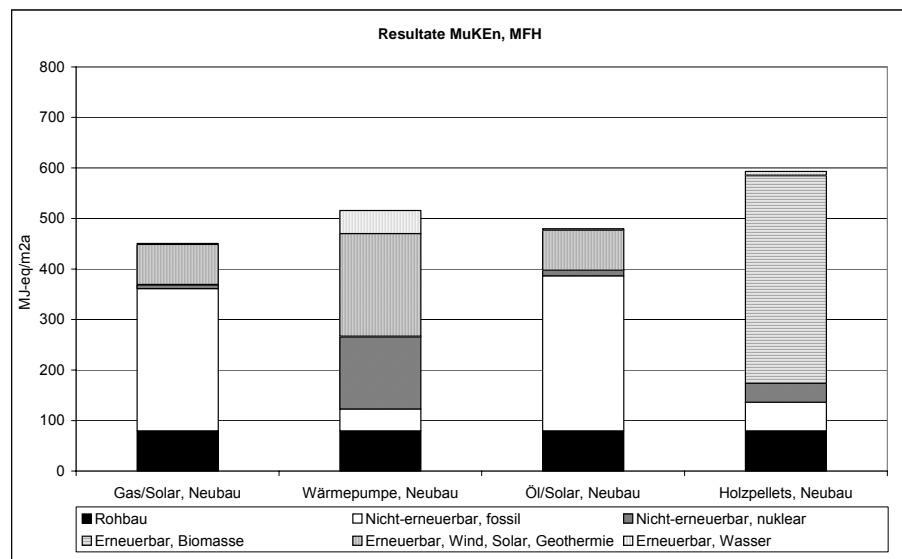
Abbildung 26: Kumulierter Energieaufwand, total (in MJ-eq/m 2 a) für Bau, Betrieb und Rückbau von Mehrfamilienhäusern nach MuKE n Modul 2 für Neubauten. Der Anteil Rohbau (ohne Wärmedämmung) ist separat ausgewiesen.
