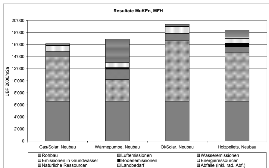
Abbildung 34: Umweltbelastungspunkte 2006/m 2 a (provisorische Ökofaktoren) für Bau, Betrieb und Rückbau von Mehrfamilienhäusern nach MuKE n Modul 2 für Neubauten. Der Anteil Rohbau (ohne Wärmedämmung) ist separat ausgewiesen.
