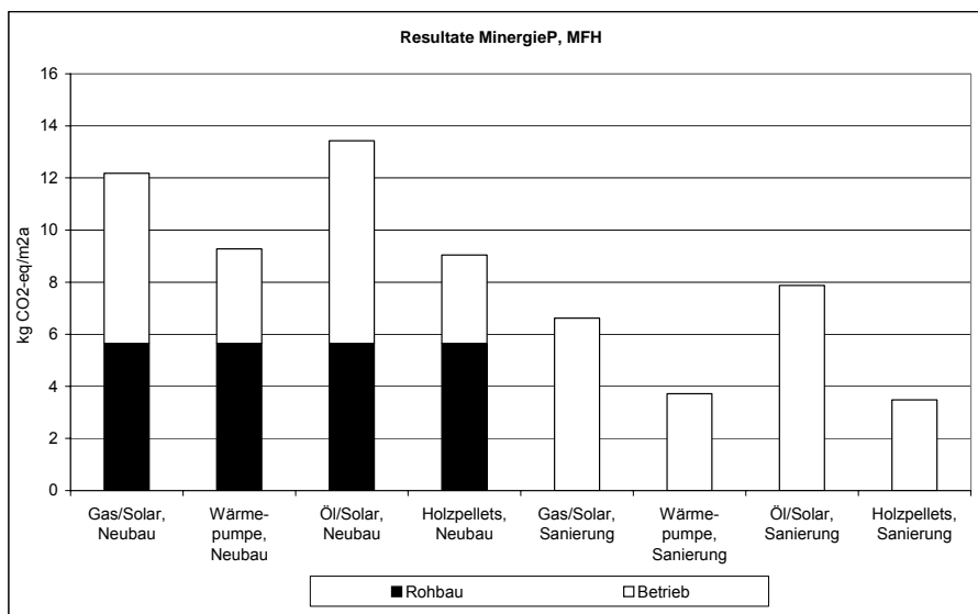
Abbildung 50: Treibhauspotential (in kg CO 2 -eq/m 2 a) für Bau, Betrieb und Rückbau von Mehrfamilienhäusern nach Minergie-P für Neubauten und Sanierungen. Der Anteil Rohbau (ohne Wärmedämmung) ist separat ausgewiesen.
