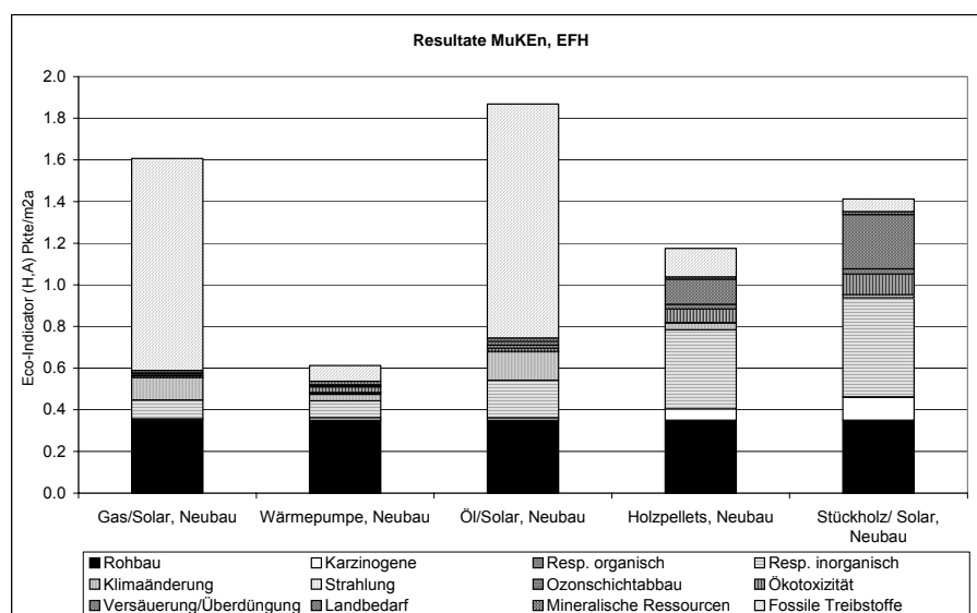
Abbildung 30: Eco-indicator '99 (H, A) Punkte/m 2 a für Bau, Betrieb und Rückbau von Einfamilienhäusern nach MuKE Modul 2 für Neubauten. Der Anteil Rohbau (ohne Wärmedämmung) ist separat ausgewiesen.
