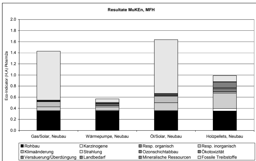
Abbildung 31: Eco-indicator '99 (H, A) Punkte/m 2 a für Bau, Betrieb und Rückbau von Mehrfamilienhäusern nach MuKEn Modul 2 für Neubauten. Der Anteil Rohbau (ohne Wärmedämmung) ist separat ausgewiesen.
