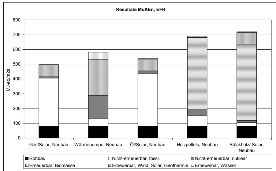
Abbildung 25: Kumulierter Energieaufwand, total (in MJ-eq/m 2 a) für Bau, Betrieb und Rückbau von Einfamilienhäusern nach MuKE n Modul 2 für Neubauten. Der Anteil Rohbau (ohne Wärmedämmung) ist separat ausgewiesen.
