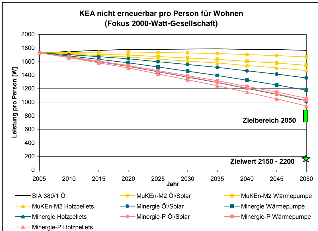
Abbildung 76 Prognose des Kumulierten Energieaufwandes nicht erneuerbar (KEA) pro Kopf für den Schweizer Wohngebäudepark bis 2050 für verschiedene Kombinationen von Baustandards und Energiesystemen. Ziele für die 2000-Watt-Gesellschaft gemäss verschiedener Autoren (siehe Kapitel 9.1.3).
