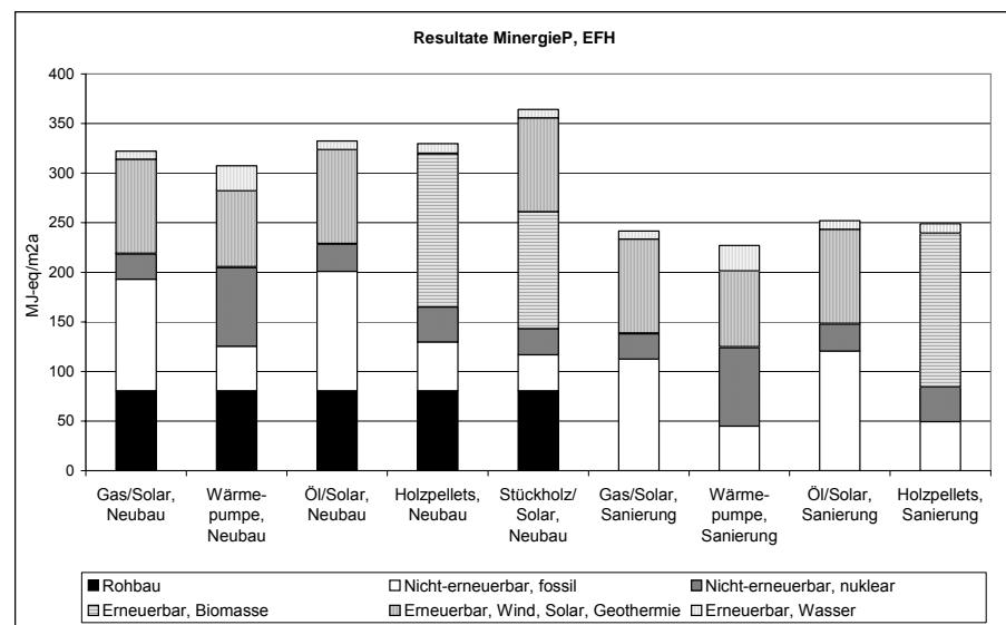
Abbildung 47: Kumulierter Energieaufwand, total (in MJ-eq/m 2 a) für Bau, Betrieb und Rückbau von Einfamilienhäusern nach Minergie-P für Neubauten und Sanierungen. Der Anteil Rohbau (ohne Wärmedämmung) ist separat ausgewiesen.
