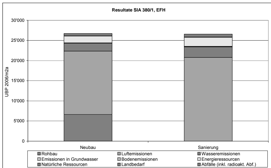
Abbildung 22: Umweltbelastungspunkte 2006/m 2 a (provisorische Ökofaktoren) für Bau, Betrieb und Rückbau von Einfamilienhäusern nach SIA 380/1 Grenzwert für Neubau bzw. Sanierung. Der Anteil Rohbau (ohne Wärmedämmung) ist separat ausgewiesen.
