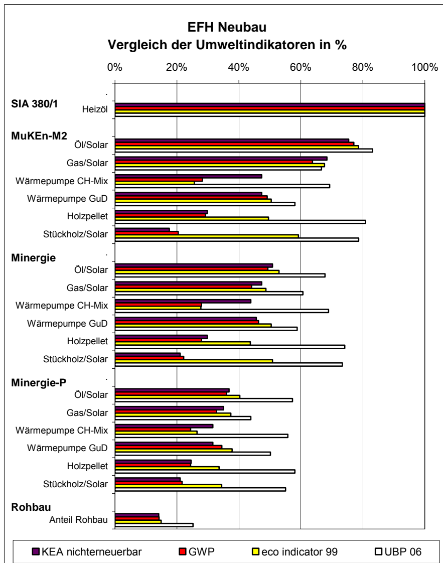
Abbildung 2: Relativer Vergleich der Resultate der unterschiedlichen Bewertungsmethoden für EFH Neubau. Bei Neubauten ist die Umweltwirkungen des Rohbaus enthalten und zur Erläuterung der Grössenordnung separat aufgeführt.
