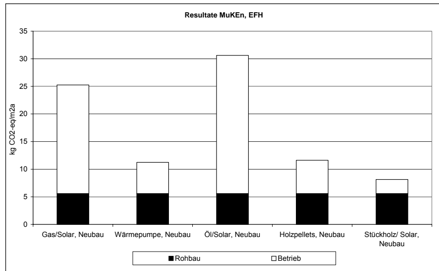
Abbildung 27: Treibhauspotential (in kg CO 2 -eq/m 2 a) für Bau, Betrieb und Rückbau von Einfamilienhäusern nach MuKE Modul 2 für Neubauten. Der Anteil Rohbau (ohne Wärmedämmung) ist separat ausgewiesen.
