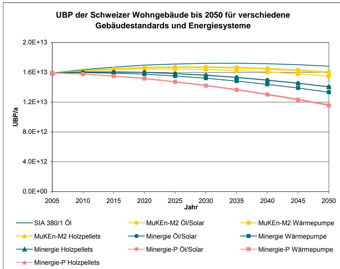
Abbildung 79 Prognose der Umweltbelastungspunkte 2006 (Methode der ökologischen Knappheit) des Schweizer Wohngebäudeparks bis 2050 für verschiedene Kombinationen von Baustandards und Energiesystemen (je Kurve alle Neubauten und Sanierungen ausschliesslich gemäss einer Kombination)
