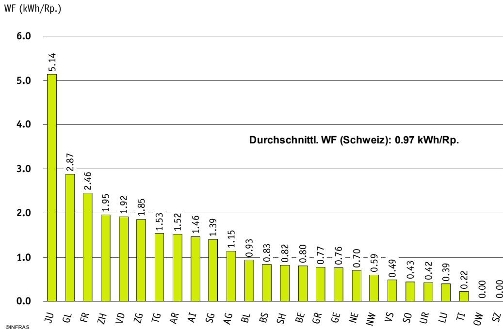
Figur 9 Wirkungsfaktoren nach Kantonen.
