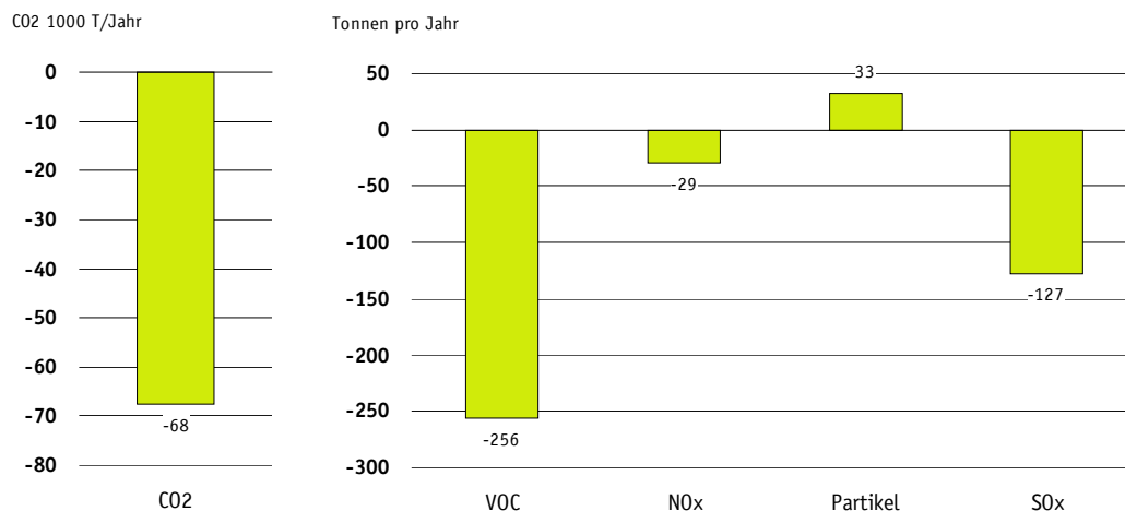
Figur 5 Auswirkungen auf CO 2 - und wichtige Schadstoffemissionen.
