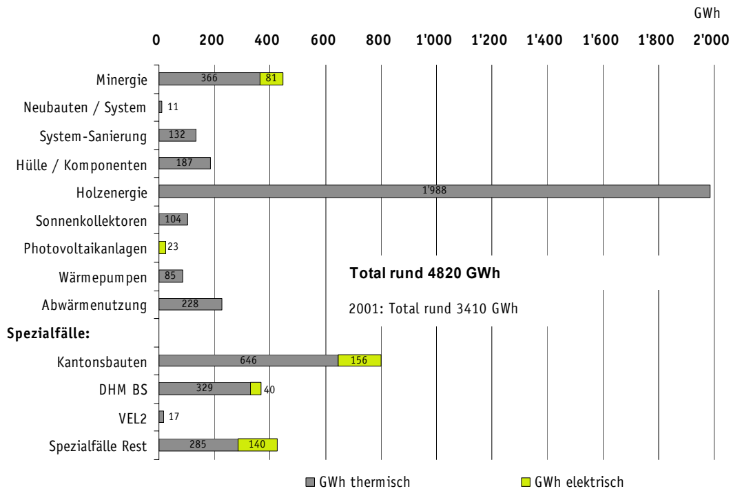
Figur 3 Ausgelöste energetische Wirkung nach Massnahmen über Lebensdauer.
