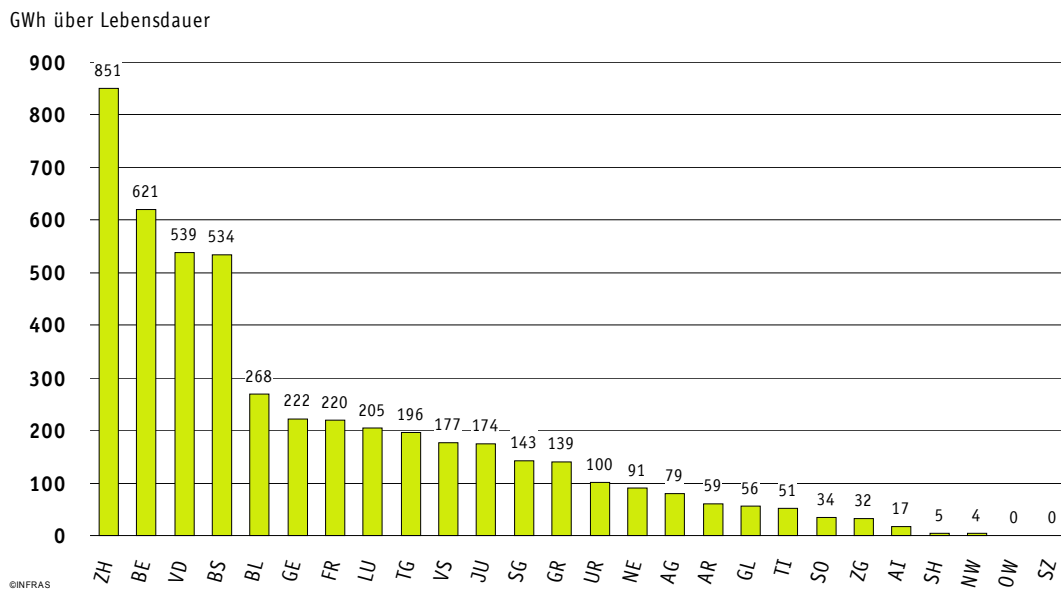
Figur 4 Energetische Wirkungen der direkten Massnahmen 2002 nach Kantonen (über Lebensdauer)
