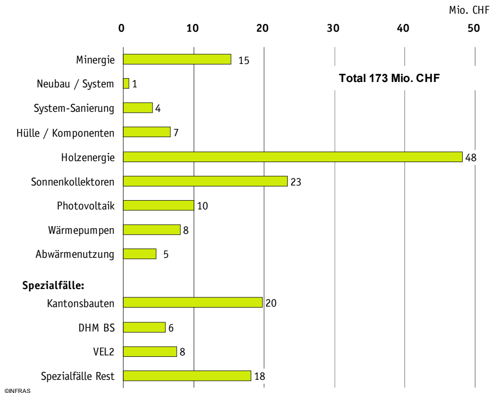
Figur 6 Ausgelöste Investitionen nach Massnahmen.
